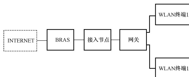
图 6 WLAN 安全性测试配置
